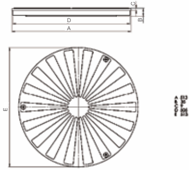
Muayene Baca Kapak Ölçüsü
